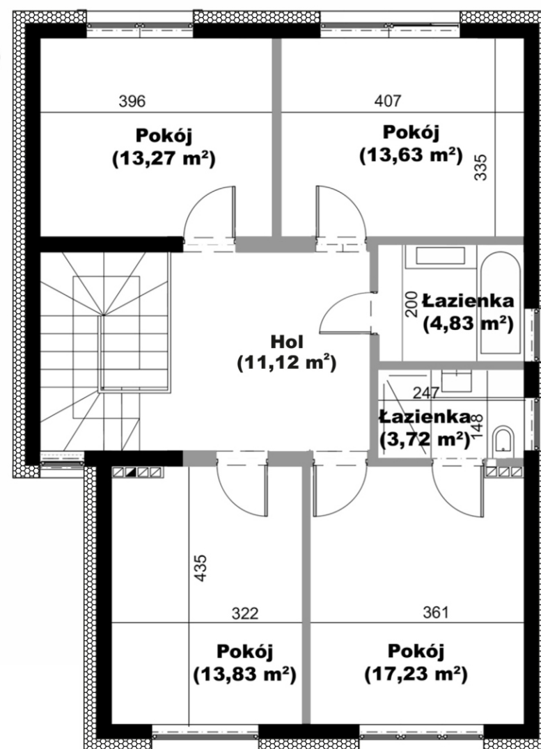
Piętro (80,61 m 2 )
